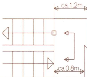
Medidas mínimas del rellano delante de la escalera de subida y bajada
